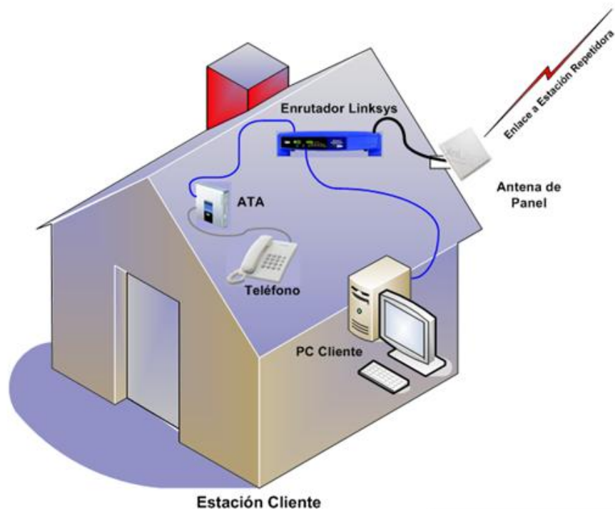
Esquema de Conexiones LAN en una Estación Cliente
